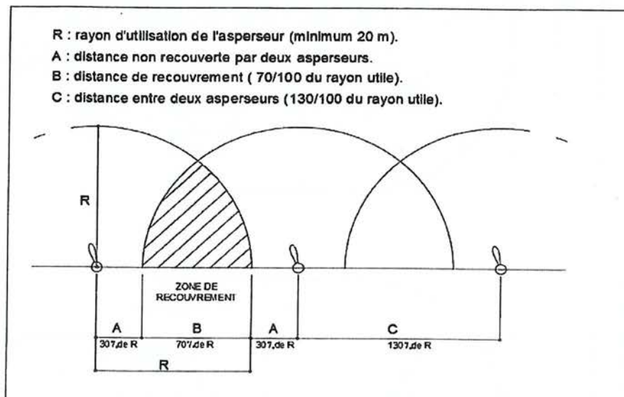
Figure 2. Schéma de principe des asperseurs (Source : SDIS06)
