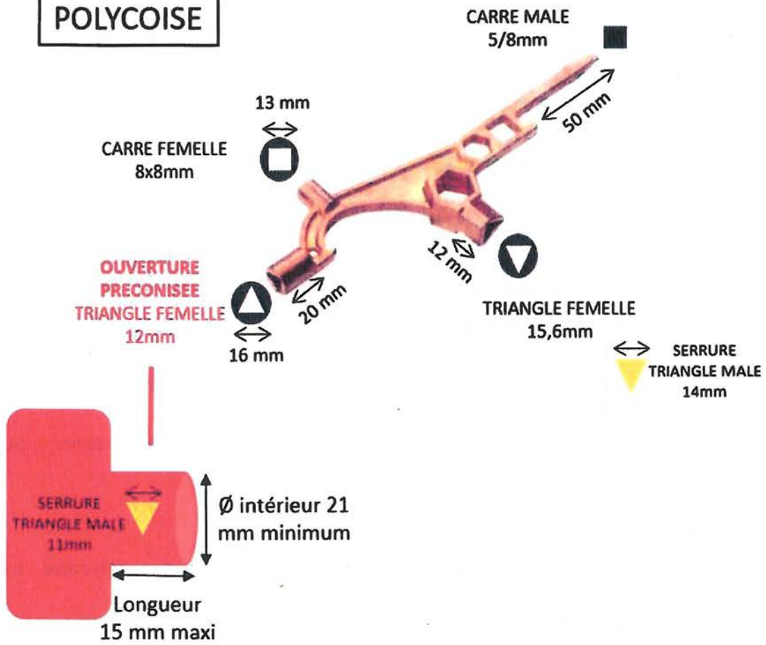
Figure 3. Caractéristiques de la clé polycoise multifonctions (Source : SDIS06)
